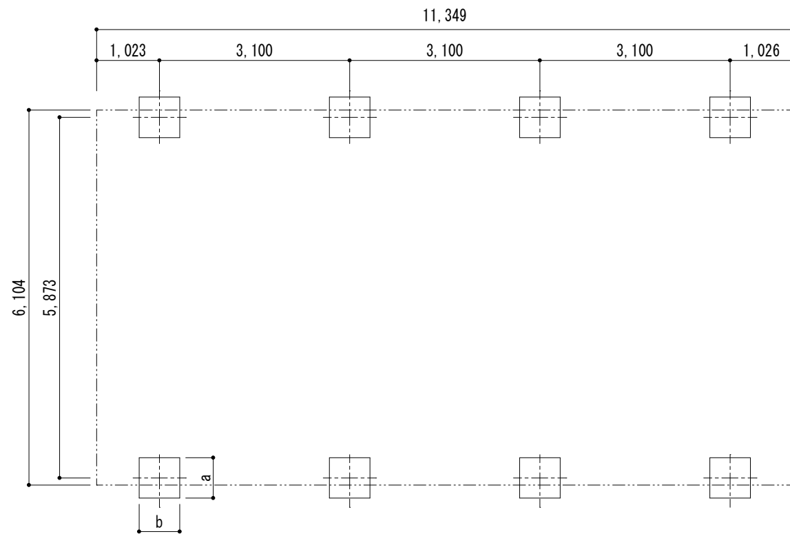
■基礎配置図
